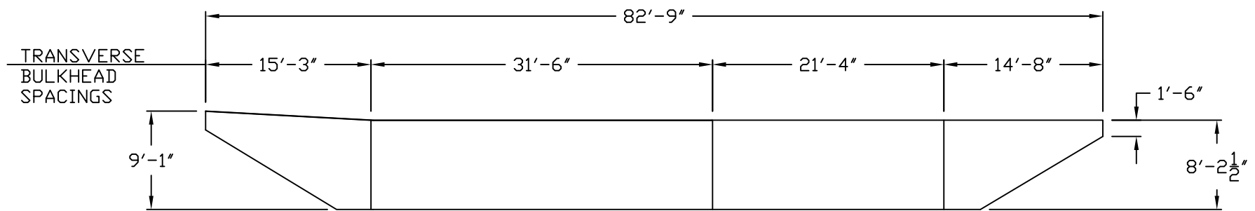
CSM 23 - Elevation
